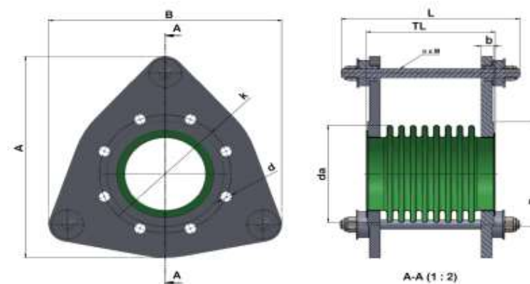
Fig. 2: Dreieckflansch
