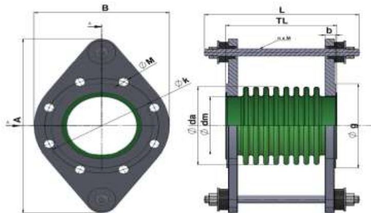
Fig. 1: Ovalflansch
