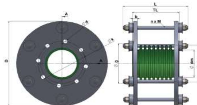
Fig. 4: Bride ronde
