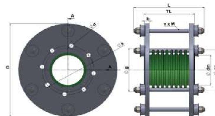
Fig. 4: Rundflansch
