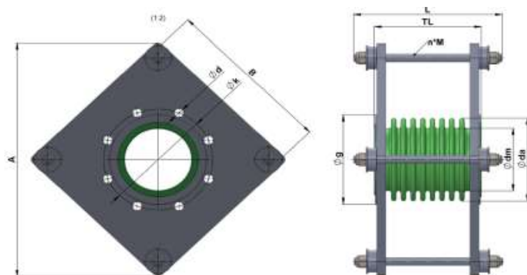
Fig. 3: Bride carrée
