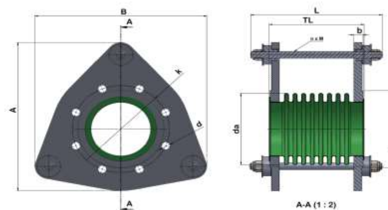
Fig. 2: Bride triangulaire
