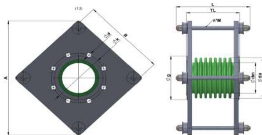
Fig. 3: Viereckflansch
