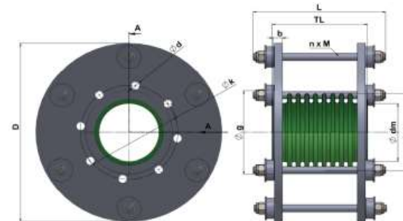
Fig. 4: Round flange
